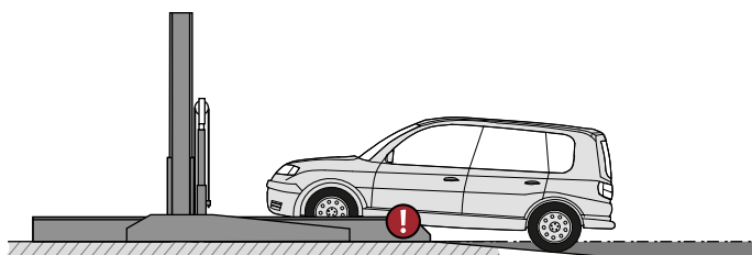
max. 14% Steigung
