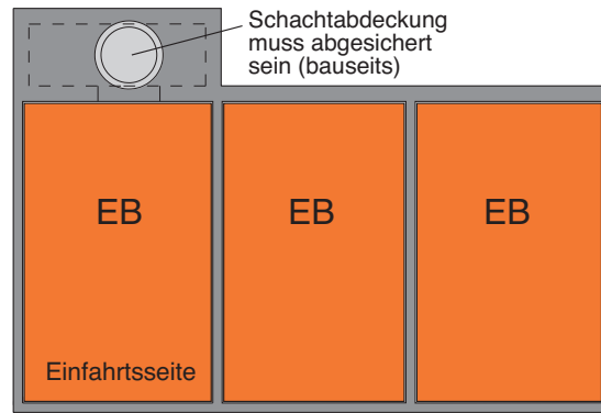
Reihenanlage (mit Zwischenwänden)
